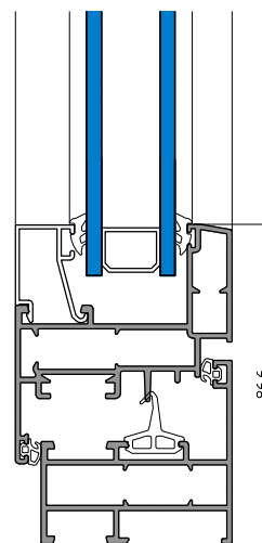
Sección Vertical
