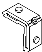
Escuadra Vta. Rpt Marco y hoja ventana REF: 82110
